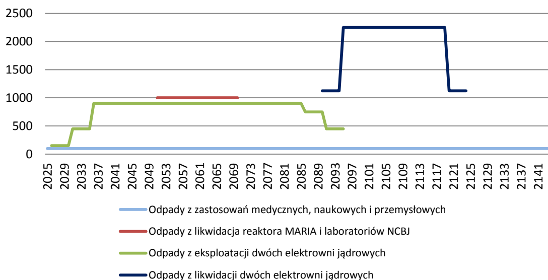
Rys. 3.5. Prognoza dostaw nisko- i średnioaktywnych odpadów promieniotwórczych do NSPOP w latach 2025 - 2144 [m 3 ]
