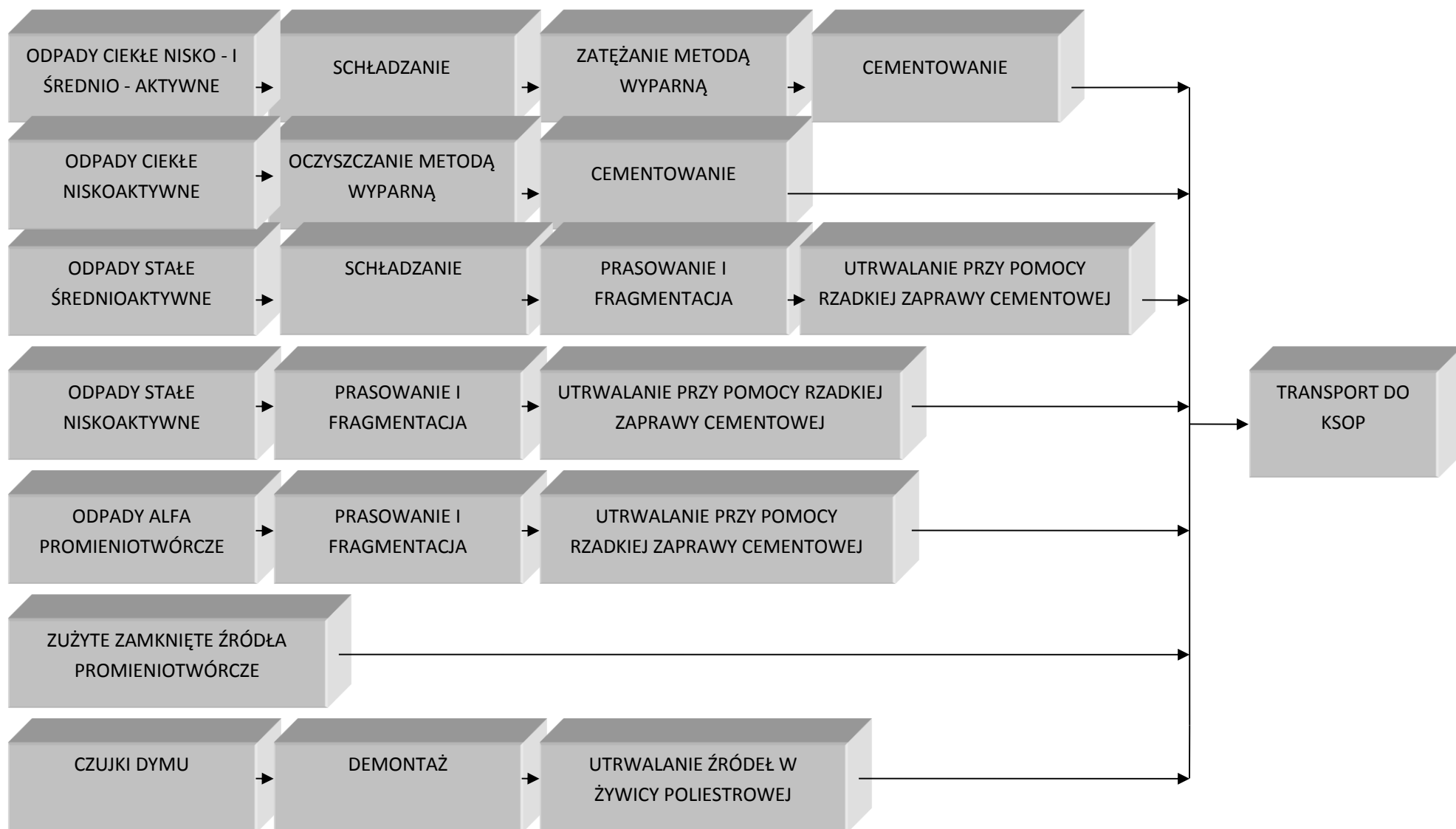
Rys. 4.1. Schemat postępowania z nisko- i średnioaktywnymi odpadami promieniotwórczymi w Polsce
