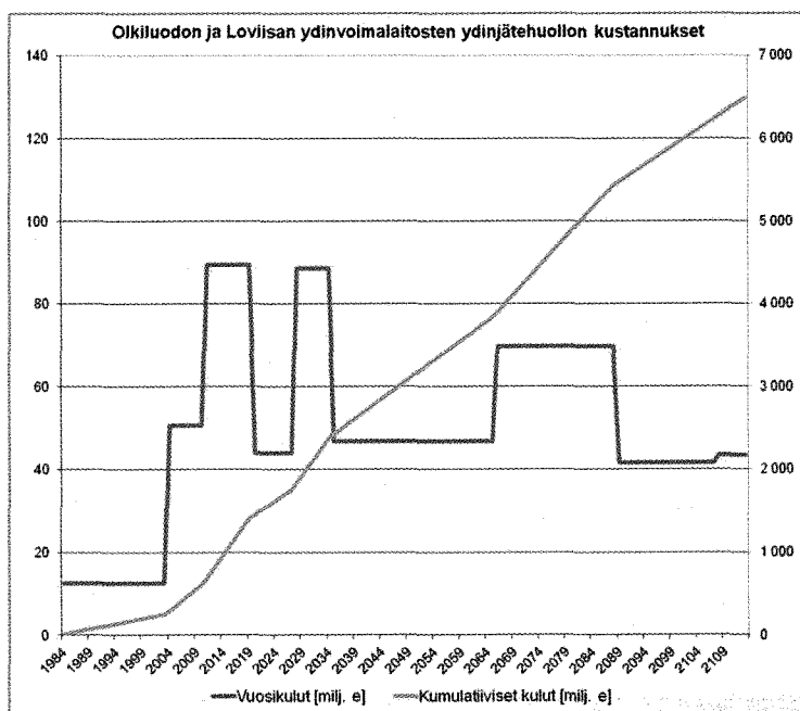
Kuva. Olkiluodon ja Loviisan ydinvoimalaitosten ydinjätehuollon kustannukset (lähde TVO).
