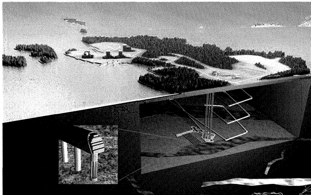
Kuva. Havainnekuva KBS-3V-loppusijoitusratkaisusta (lähde: Posiva).
